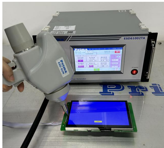
图 5-2 ESD 测试图
