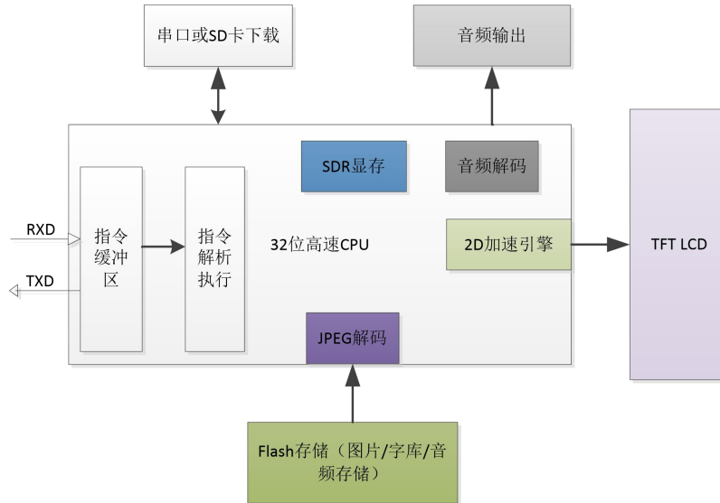
图 9-1 HMI 硬件结构参考图
